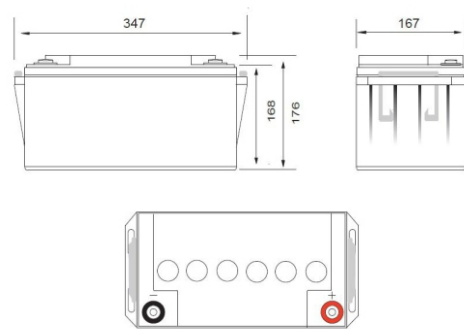
Wymiary
