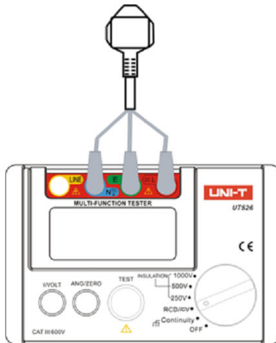
Rysunek 3. Schemat połączeń do testowania wyłączników różnicowoprądowych.
