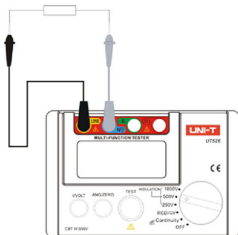
Rysunek 5. Pomiar rezystancji izolacji
