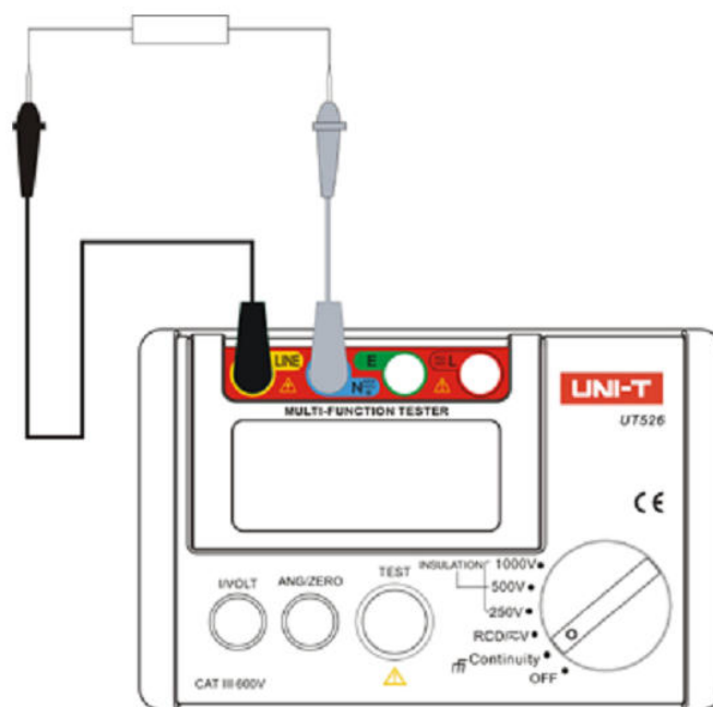
Rysunek 2. Schemat połączeń do pomiaru rezystancji pętli linii (uziemienia)
