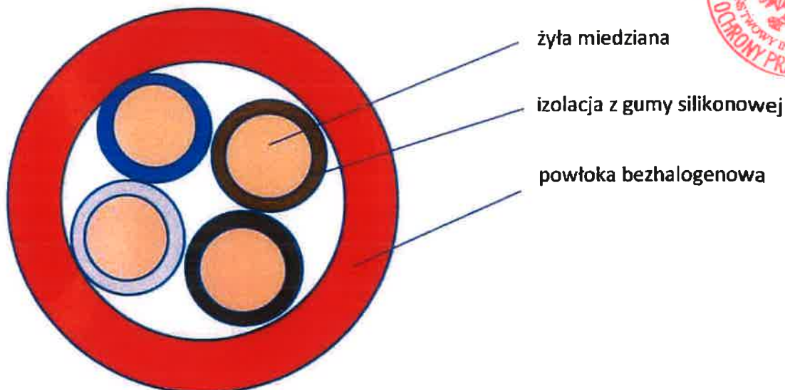
Rys. 1. Budowa kabla typu HDGs FE180/PH120/E90 Źródło: Materiały producenta.
