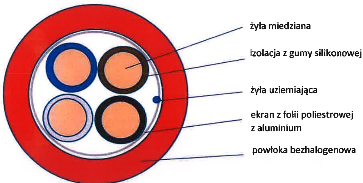
Rys. 2. Budowa kabla typu HDGsekwf FE180/PH120/E90 Źródło: Materiały producenta.
