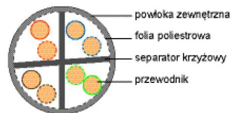
Kabel Kat6 U/UTP
