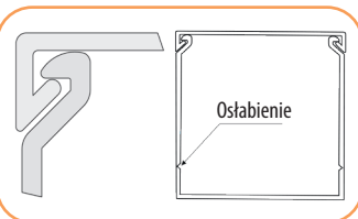
Zapięcie pokrywy - typ B
