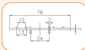
Profil płaski UPO CP
