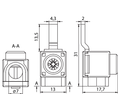
EFB-25PT-15
