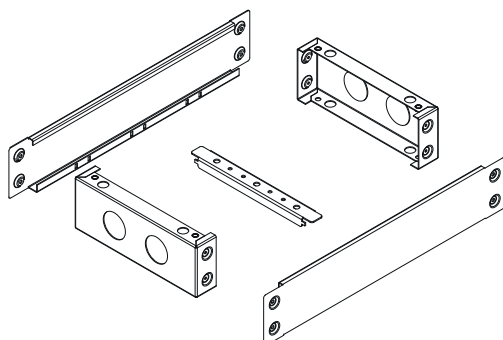
4-elementowy cokół z poprzeczką do mocowania przewodów i kabli
