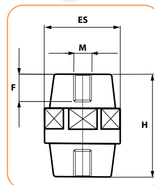
F-głębokość gwintu tulejki
