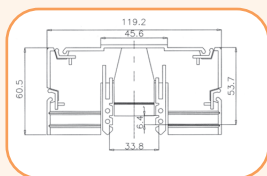
Nośnik UPO TP
