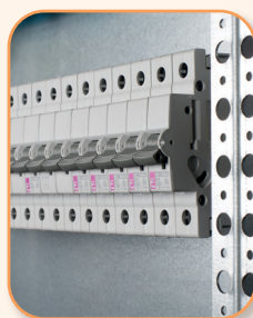
Aparatura modułowa
