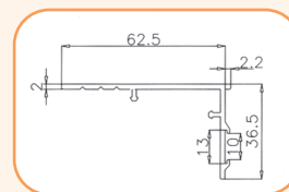
Profil kątowny UPO FP
