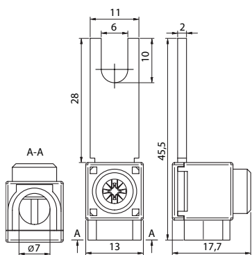
EFB-25FT-28
