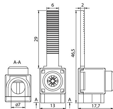
EFB-25PT-29
