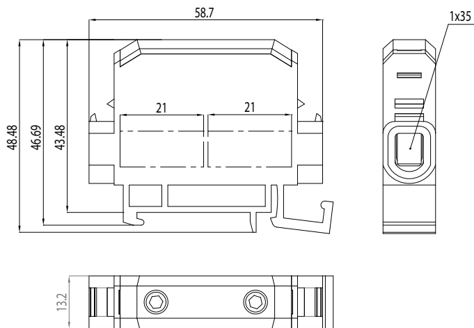
EDBJ-1x35-1x35
