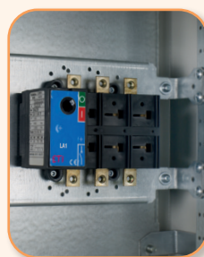
Rozłącznik LA 1 160 A
